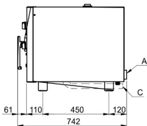
Vue côté
